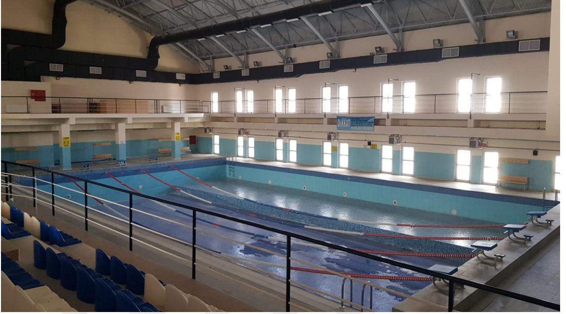
Fotoğraf 5.13. İsmail Eren Spor Tesisi - Yarı Olimpik Yüzme Havuzu (2023)
