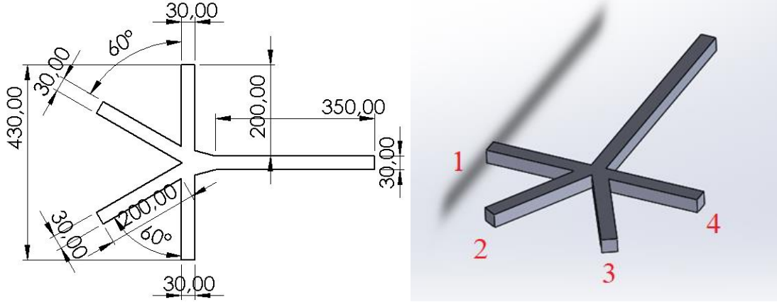
Şekil 1. 4 kanallı mikro-akışkanın teknik resmi ve 3B tasarımı.
